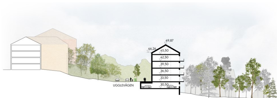
Figur 9: Längdsektion genom Ugglevägen och den föreslagna bebyggelsen. Illustration: Bergkrantz arkitektur.
