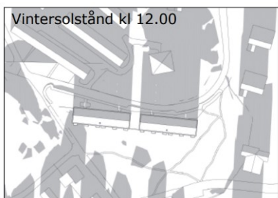
Figur 16: Solstudie för nya bostäders påverkan på befintliga bostäder. Fullständig solstudie finns i gestaltungsprogrammet. Illustration: Bergekrantz arkitektur
